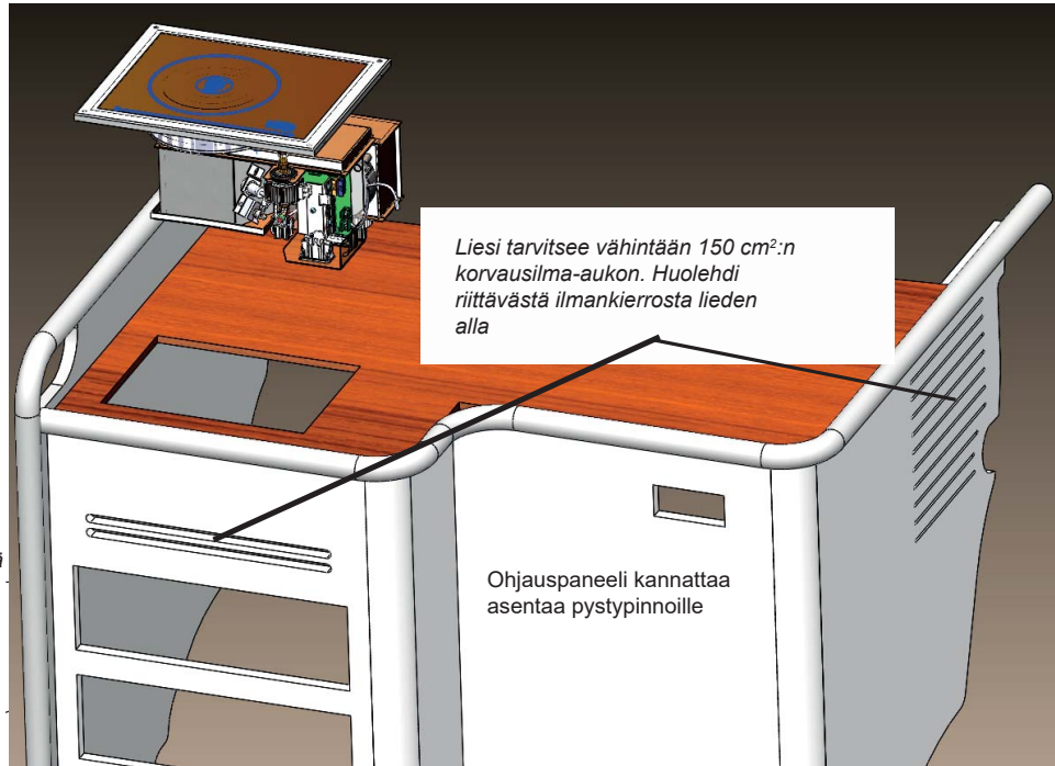
Laitteen mitat
