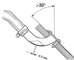
Peräpeiliin asennus
