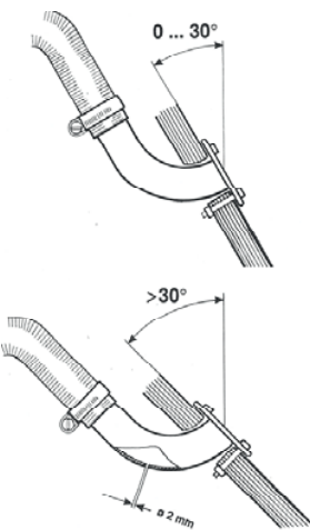
Installering i akterspegeln
