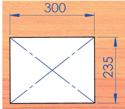
Asennusreijän koko.
