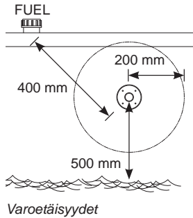
Varoetäisyydet
